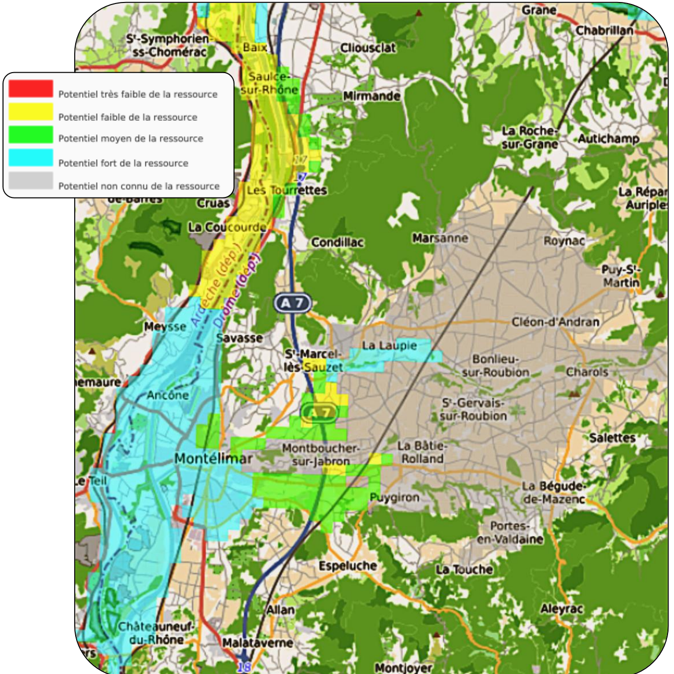
Ressources géothermiques de surface sur système ouvert (nappe) Montélimar Agglomération
